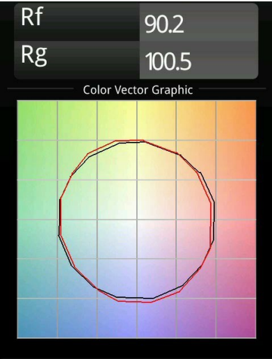
TM30 & CRI Diagramm
