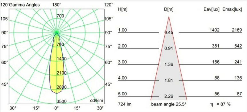
Lichtverteilung und Lichtverteilungskurve
